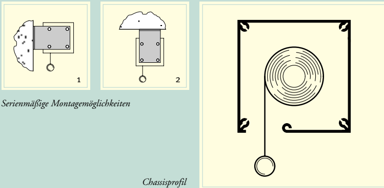
Chassisprofil
